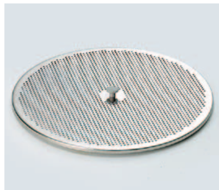
Deckel aus CrNi-Stahl, runde Lochung Ø 4 mm
